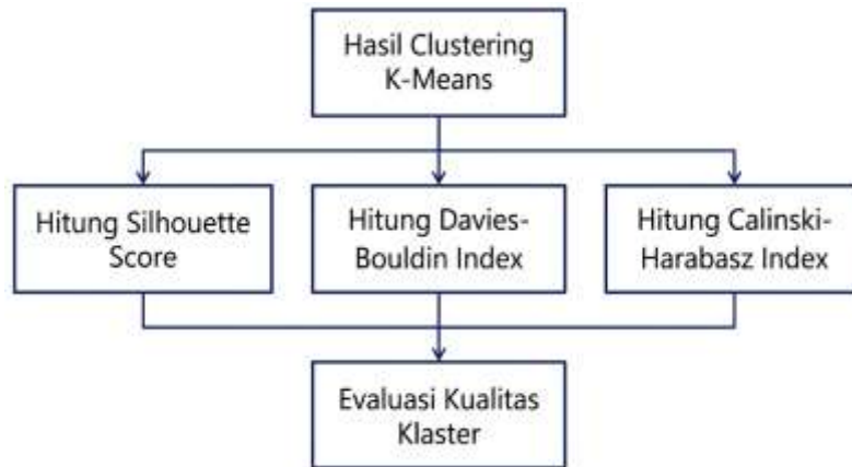
Gambar 3.4 Diagram Alir Perhitungan Metrik Evaluasi Kuantitatif Clustering
